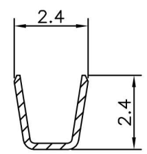
A-A SEC
